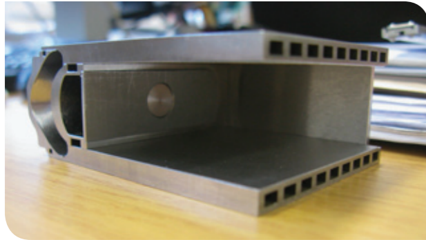
Schnitt durch Kühlplatte der Breeder-Units
