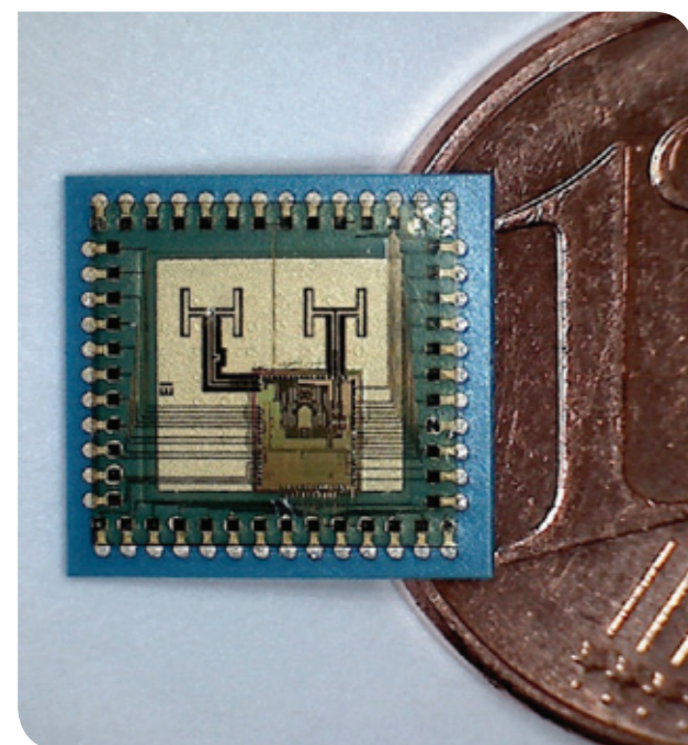
Radarsystem auf einem Chip
